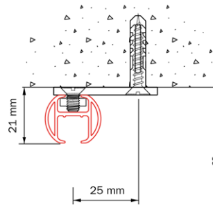
Deckenmontage 4200 mit Deckenträger 5135
