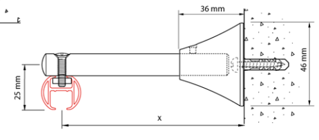
Wandmontage mit kürzbarem Wandwinkel 4217-101, der Wandwinkel kann auf x = 50 mm gekürzt werden
