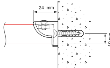
Wandmontage 4200 mit Lagerträger 4249
